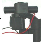
Wasserventil Fußraumheizung für S400, O350, O580, Vergl.-Nr. A0028305684 € 169,50 Art.-Nr. 1,10,30,03,024
